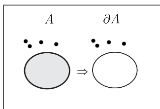
Рис. 25. Граница множества A .
