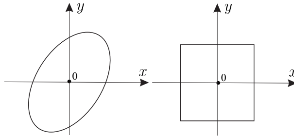
Рис. 34. Уравновешенные множества в \mathbb{R}^2 при \lambda \in [-1, 1] .
