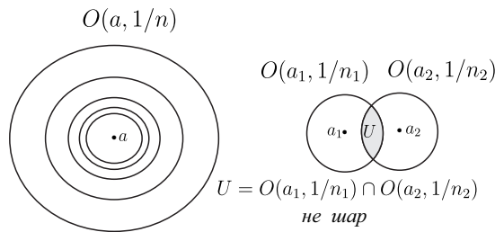
Рис. 21. Локальные базы не образуют топологии.
