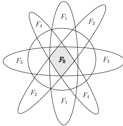
Рис. 14. Центрированная система множеств.
