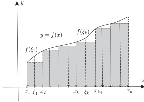
Рис. 1. Построение интегральной суммы.
