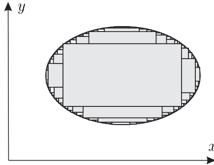
Рис. 6. Покрывание множества прямоугольниками.
