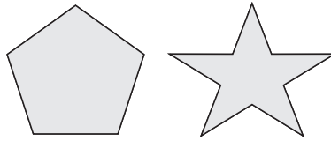
Рис. 33. Выпуклое и не выпуклое множества.
