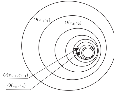
Рис. 20. Система вложенных шаров.
