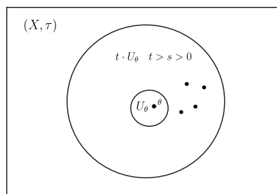
Рис. 36. Конечное число точек — ограниченное множество.
