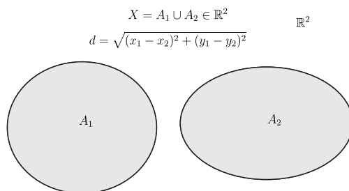
Рис. 10. Несвязное метрическое пространство.
