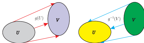
Рис. 12. Образ и прообраз множества.
