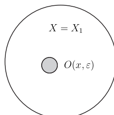
Рис. 17. Случай X = X_1 .
