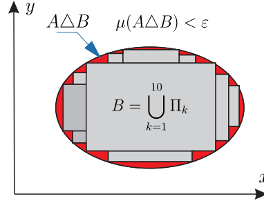
Рис. 7. « \epsilon -приближение» множества A элементарным множеством B .
