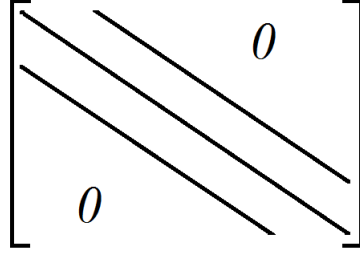
Рис. 3: Структура трехдиагональной матрицы
