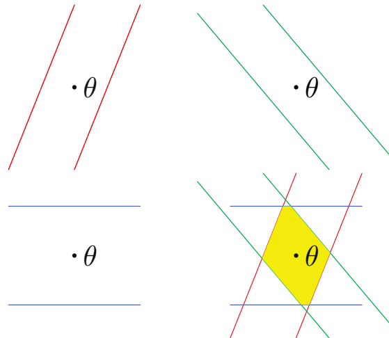
Рис. 2. Окрестность нуля как пересечение конечного числа множества вида (4.1)
