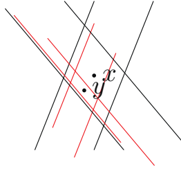
Рис. 4. Выбор окрестности, принадлежащей локальной базе \nu_y и целиком содержащейся в U_x , для некоторой точки y \in U_x
